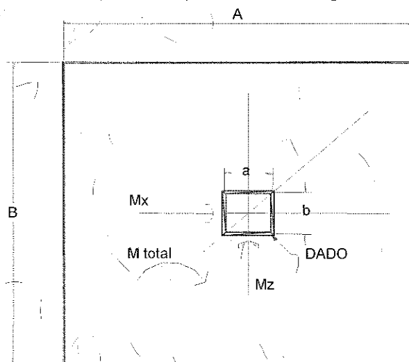
DESCOMPOSICIÓN DEL MOMENTO A APLICAR PARA REVISIÓN POR CAPACIDAD DE CARGA EN MONOPOLOS
